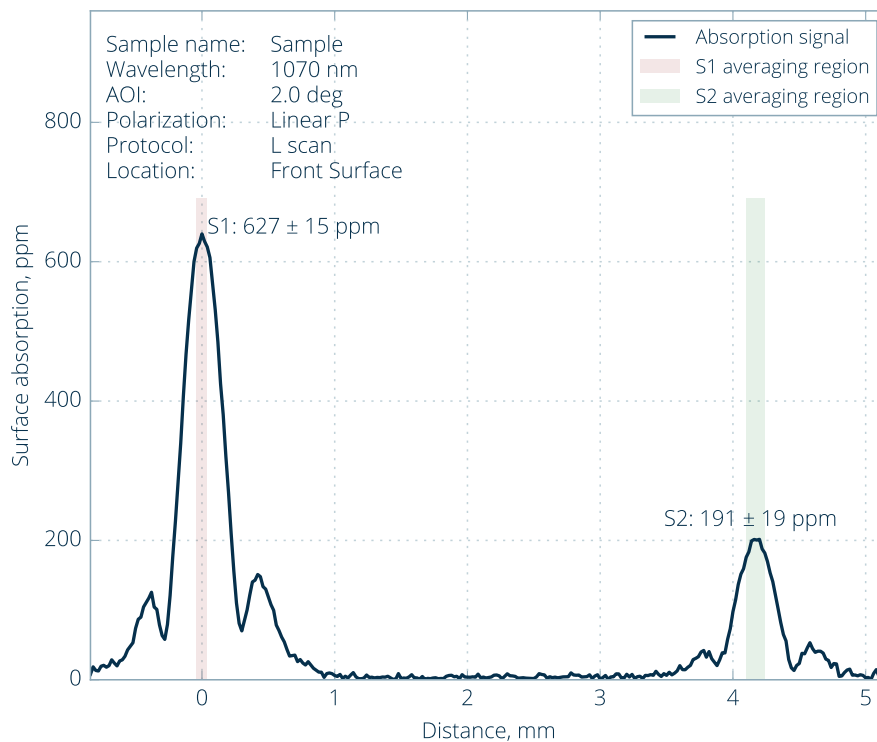
Figure 1. Longitudinal scan.
